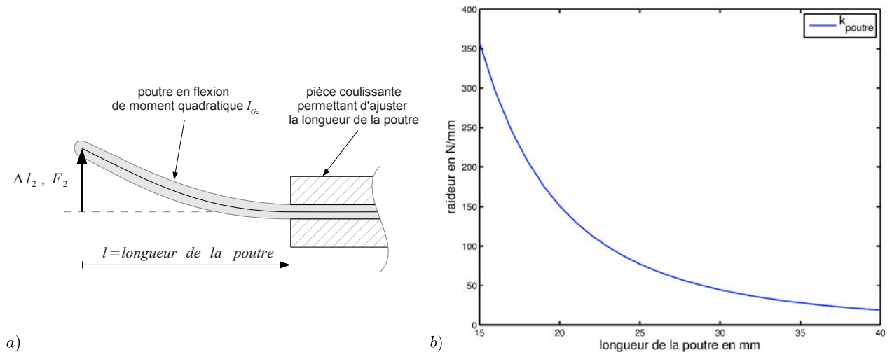
FIGURE A.3 – Principe de la raideur variable réalisé à l'aide d'une poutre en flexion. (a) schéma de la poutre de longueur variable soumise à un effort F_2 . (b) raideur de la poutre en fonction de sa longueur.
