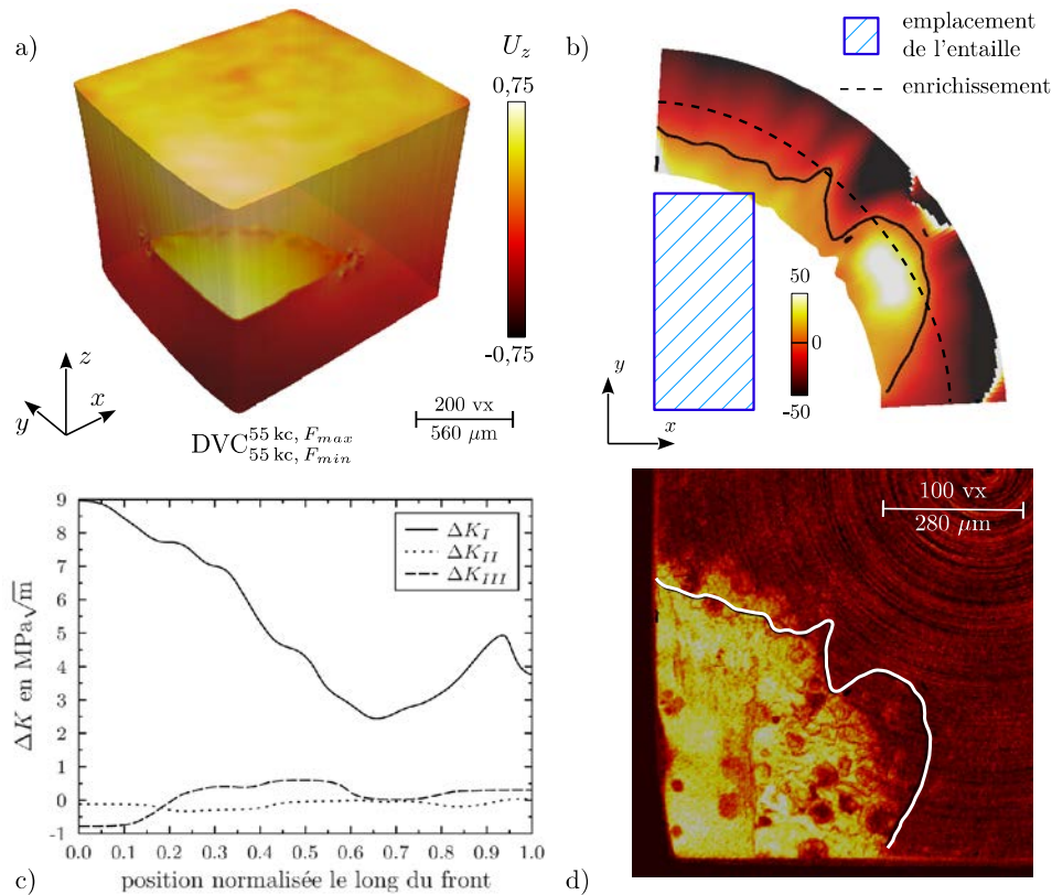
FIGURE 5.24 – Résumé des résultats pour LBj2 après 55 kc. (a) champ de déplacement et carte d'ouverture pour une régularisation utilisant une longueur d'onde de 256 \text{ vx} . (b) décalage au front (en voxel) détecté à l'aide de K_I . (c) valeurs des FICs le long du front. (d) comparaison entre le front détecté et la projection des résidus.
