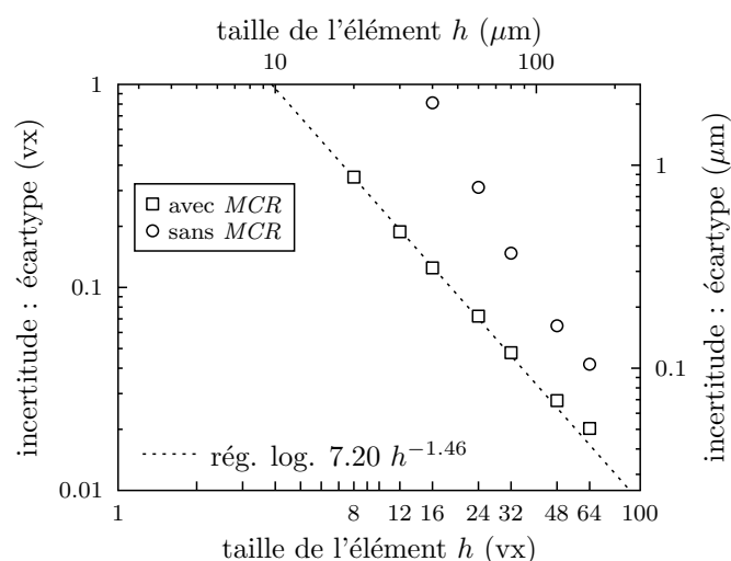
FIGURE 3.6 – Incertitude en fonction de la taille des éléments du maillage avec et sans l'utilisation de la méthode MCR . (1 vx = 2,5 μm)
