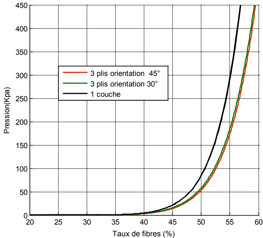
Figure 3.10 : Comparaison entre la compression d'un mono-ply et celle des multi-plis avec rotation
