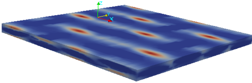
Figure 4.14 : Champ de vitesse dans la direction X d'un mono-ply à 30% de taux de fibres - Région Brinkman en bleu et Région Stokes en rouge.
