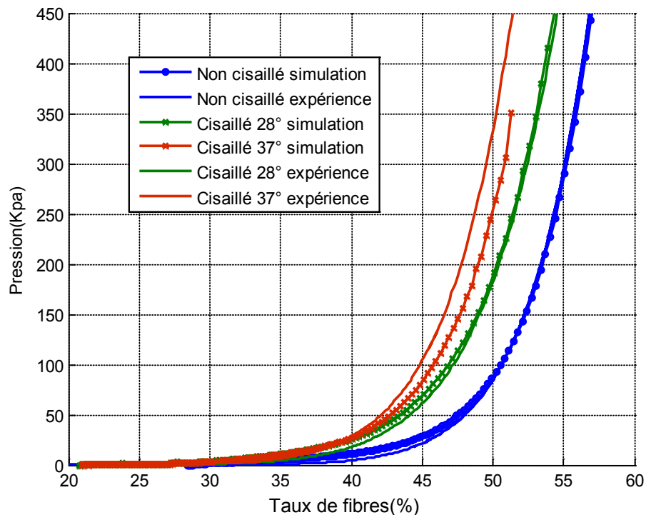
Figure 3.36 : Compression du renfort cisaillé
