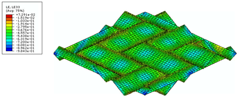
Modèle déformé (déformation \epsilon_{33} )-Cisaillement 28^\circ
