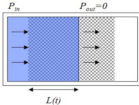
Figure 2.36 : La mesure de la perméabilité lors d'un écoulement en milieu insaturé ou en régime transitoire
