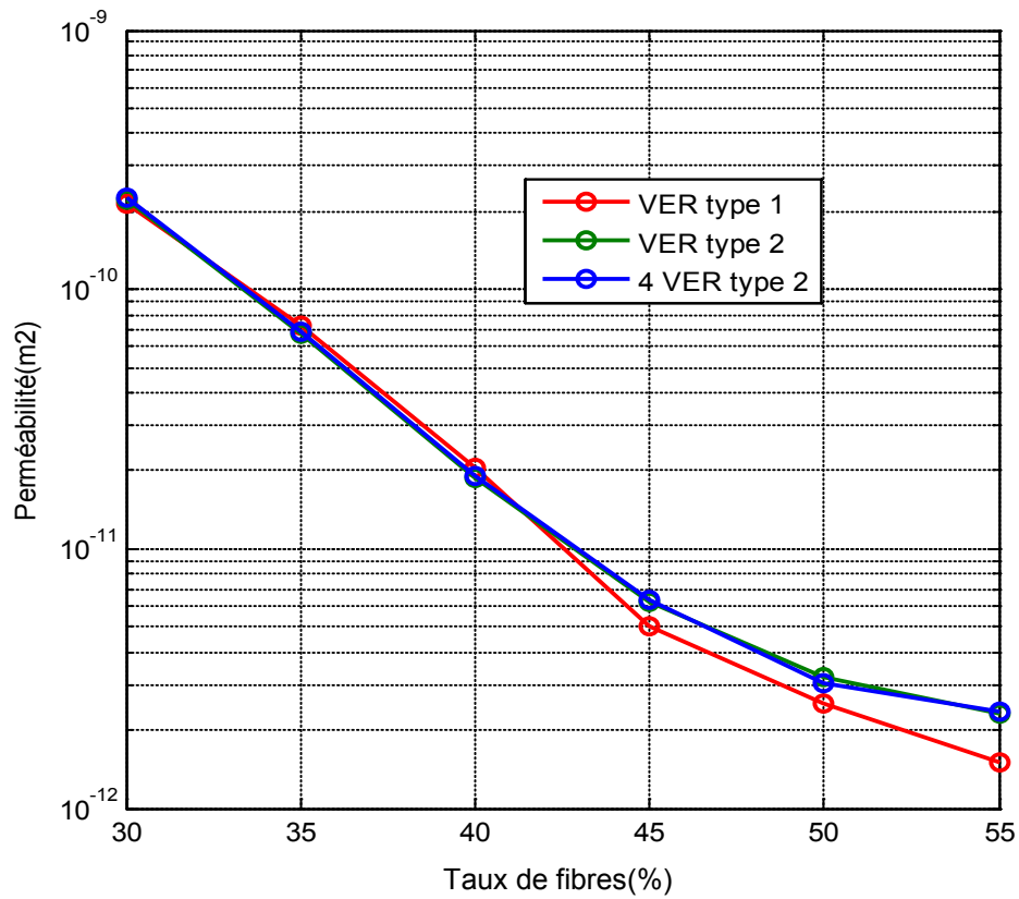
Perméabilité transverse de différents types de VER
