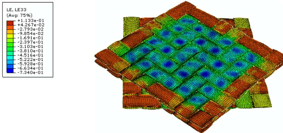
Modèle déformé (déformation \varepsilon_{33} )
