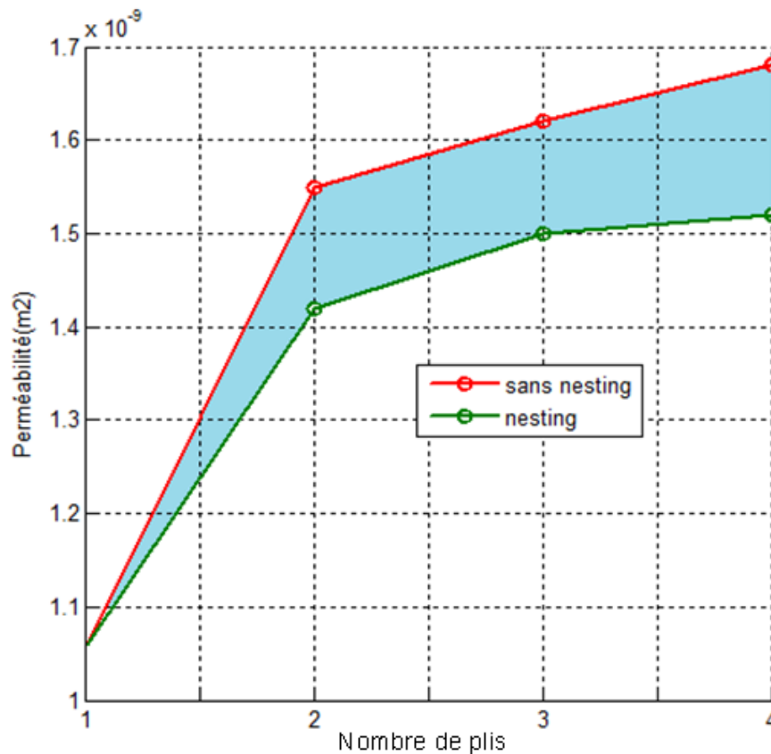
Perméabilité dans le plan des multi-plis sans nesting et avec nesting du renfort non comprimé
