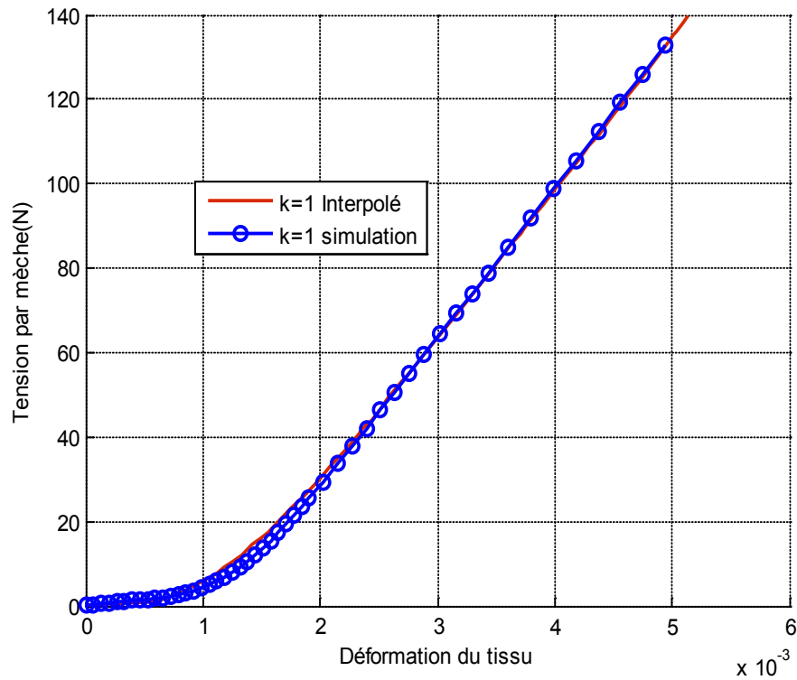
Figure 3.19 : Indentification des paramètres de matériaux
