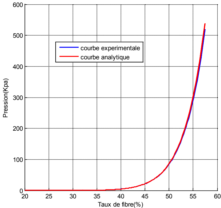
Figure 3.2 : Compression d'un pli
