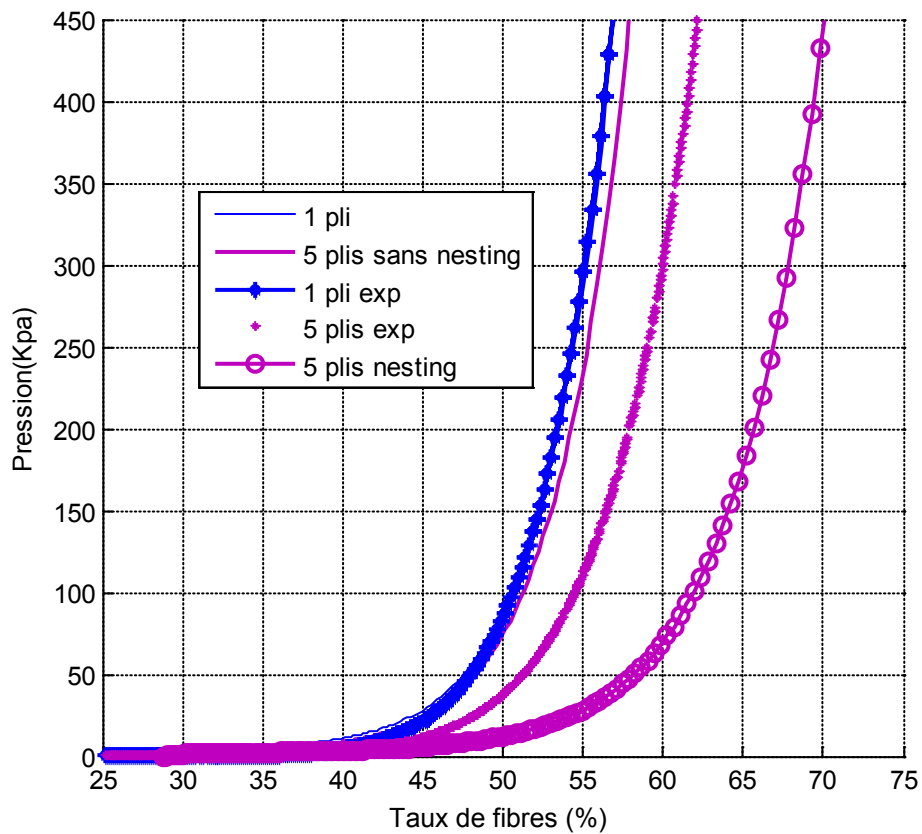
Figure 3.31 : Compression cinq plis avec nesting et sans nesting
