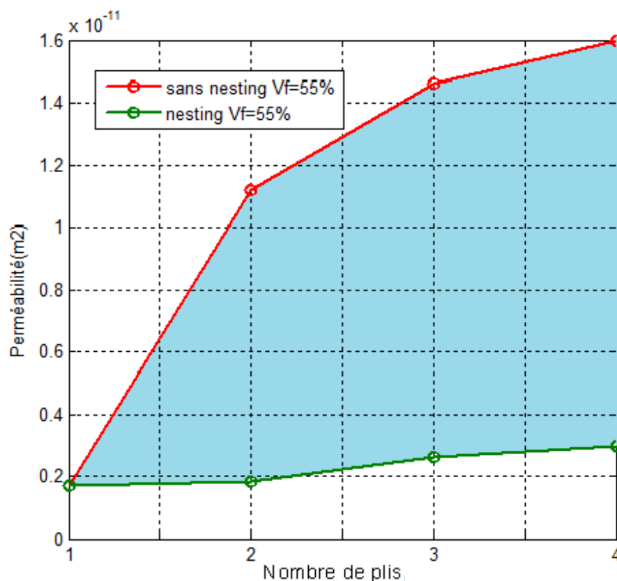
Perméabilité transverse des multi-plis sans nesting et avec nesting du renfort comprimé
