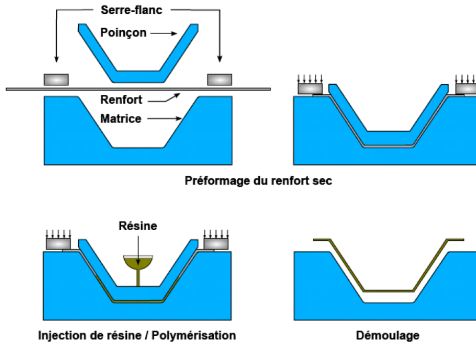
Figure 2.5 : Procédé RTM
