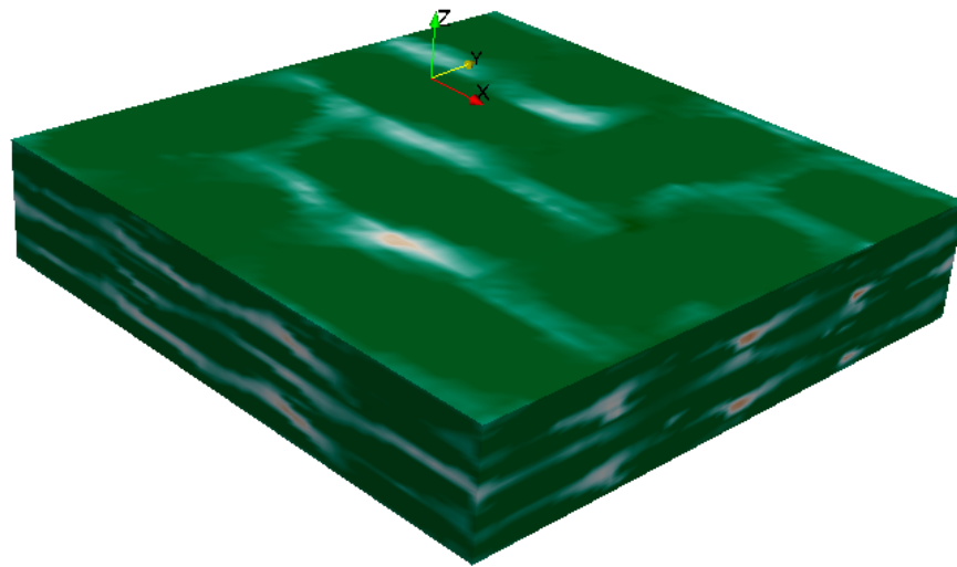
Figure 4.19 : Champ de vitesse dans la direction X de 4 plis sans nesting
