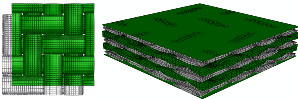
Figure 3.27 : Nesting de deux plis
