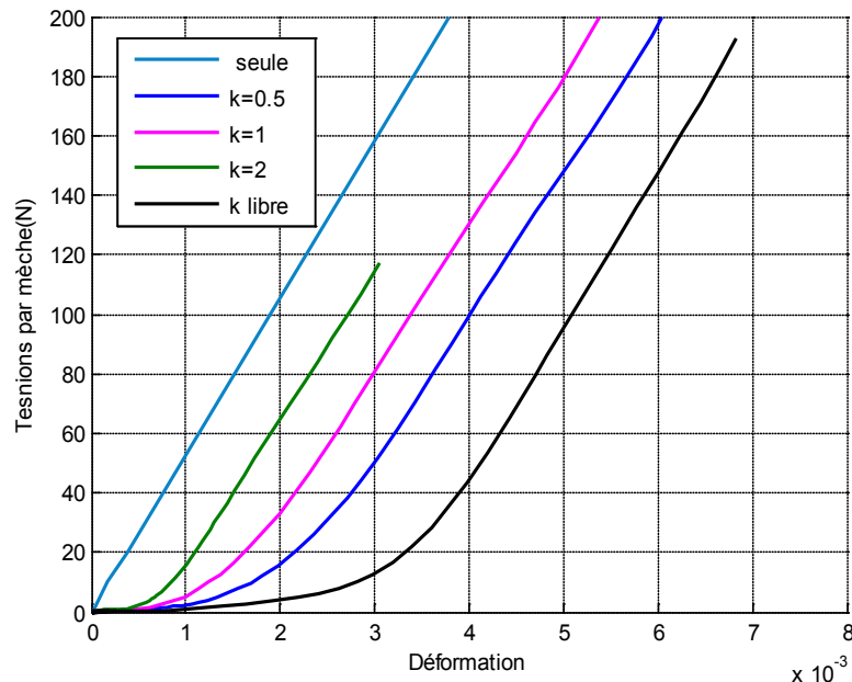
Figure 2.14 : Résultat des essais de tension biaxiale [BUE98]
