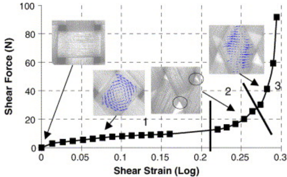
Figure 2.18 Courbe de cisaillement «Bias test » et phénomènes mésoscopiques [DUM03]
