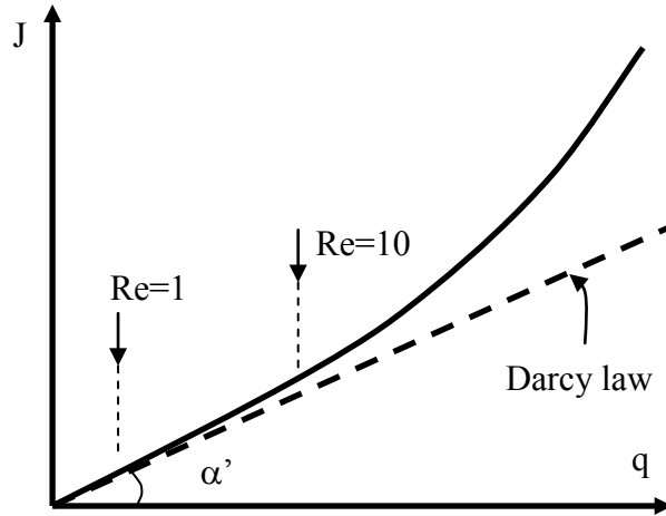
Figure 2.34: Ecoulement à travers un milieu poreux : régimes hydrauliques [BEA72]
