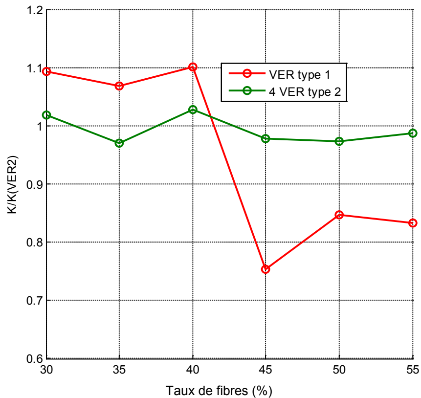
Figure 4.16 : Influence du choix de VER sur la perméabilité dans le plan
