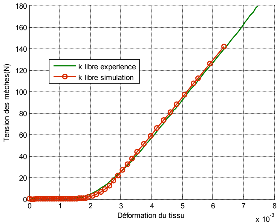
Figure 3.19 : Indentification des paramètres de matériaux
